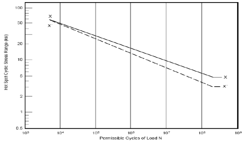
Gambar 2. Kurva S-N API untuk Analisis Kelelahan
