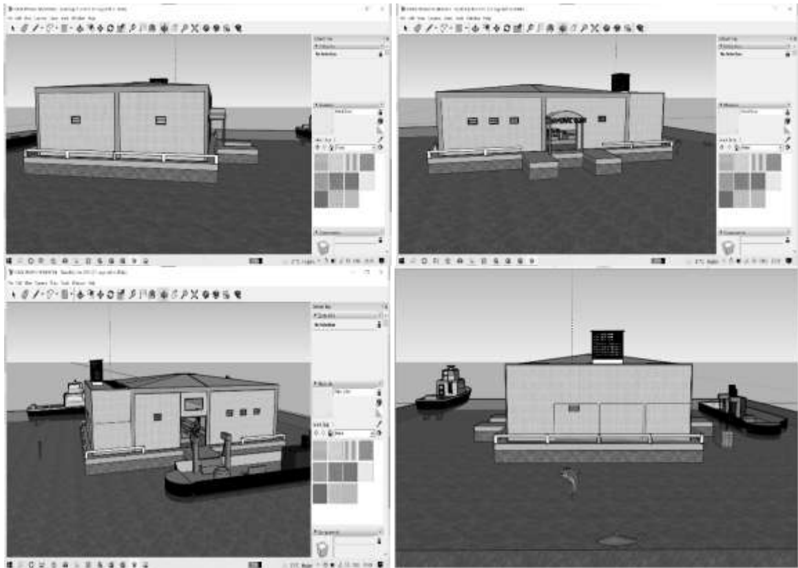
Gambar 1. Desain Terminal Ikan Terapung 3d Menggunakan Software Sketchup
