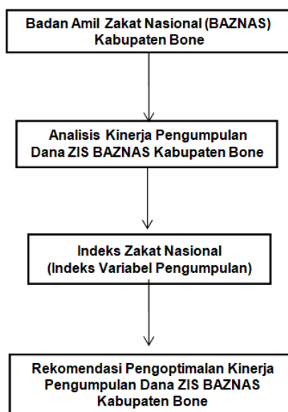
Gambar 2 Kerangka Konseptual
