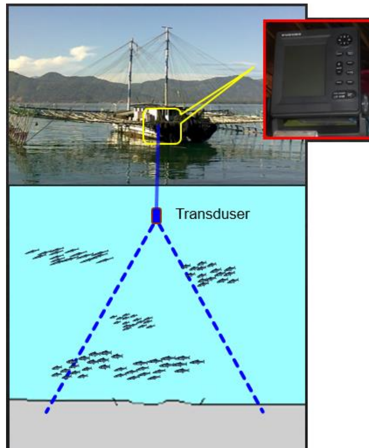
Gambar 1. Ilustrasi pemasangan echosounder pada bagan perahu
