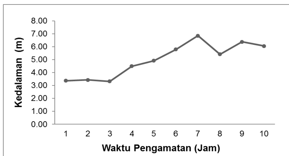
Gambar 3. Hasil pengamatan echosounder terhadap waktu kedatangan ikan
