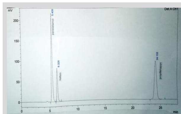
Gambar 1. Kromatogram pemisahan parasetamol, kafein dan propifenazon dengan fase gerak metanol-air pH 3 (50:50), \lambda 273 nm, laju alir 0,6 mL/menit
