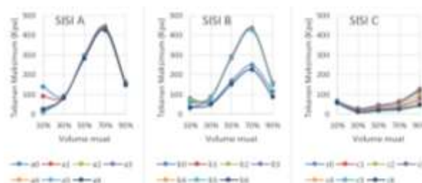
Gambar 5. Grafik tekanan maksimum terhadap volume muat frekuensi 2,145
