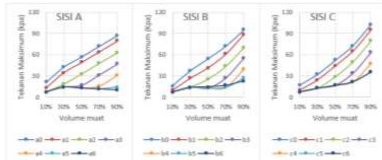
Gambar 3. Grafik tekanan maksimum terhadap volume muat
