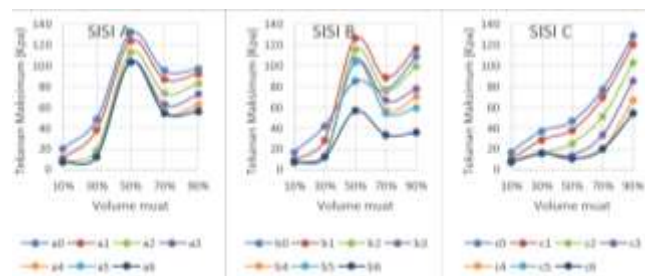
Gambar 4. Grafik tekanan maksimum terhadap volume muat frekuensi 1,43
