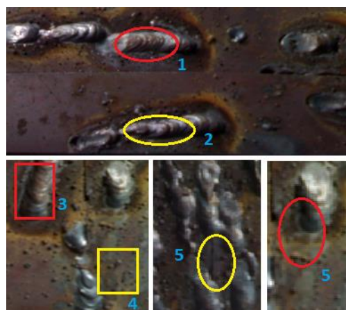
Gambar 5. Evaluasi hasil pengelasan
