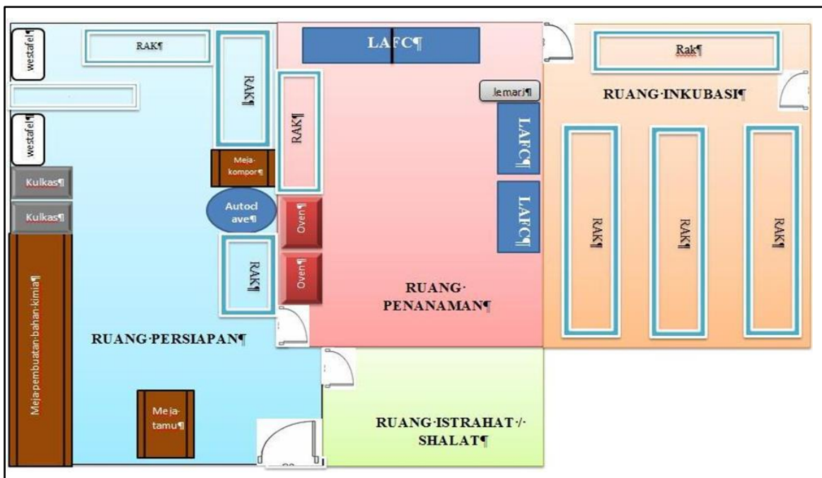
Gambar 2. Lay-out Peralatan yang sudah dimiliki dalam ruang calon PPUPIK Perbenihan Kultur Jaringan Anggrek pada Teaching Industry .
